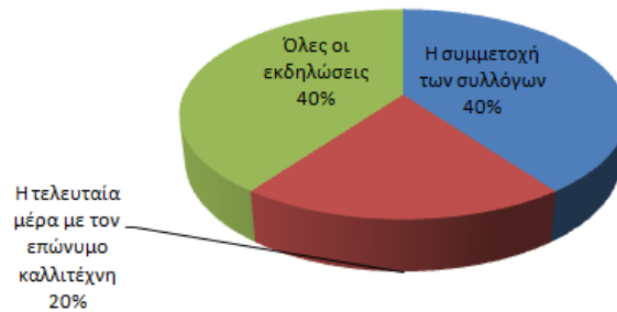
Γράφημα 2.
