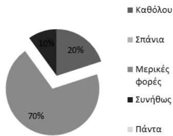
Γράφημα 2. Αγωνία
