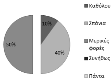
Γράφημα 1. Φόβος
