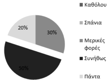
Γράφημα 4. Αισιοδοξία
