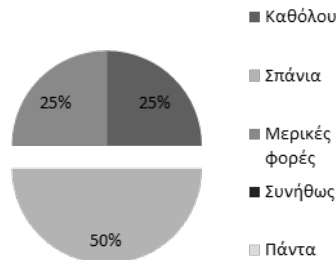
Γράφημα 3. Θυμός
