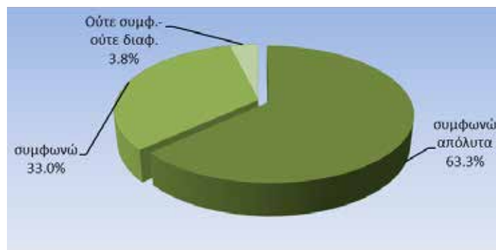
Σχήμα 3. Αναγκαιότητα ανακύκλωσης.
