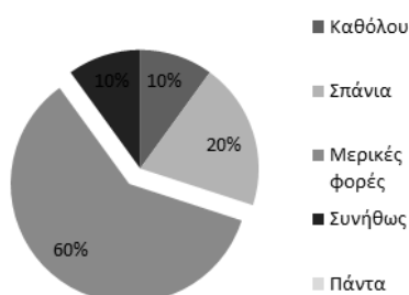
Γράφημα 6. Άγχος
