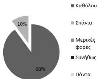
Γράφημα 5. Αδιαφορία
