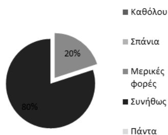
Γράφημα 7. Ικανοποίηση
