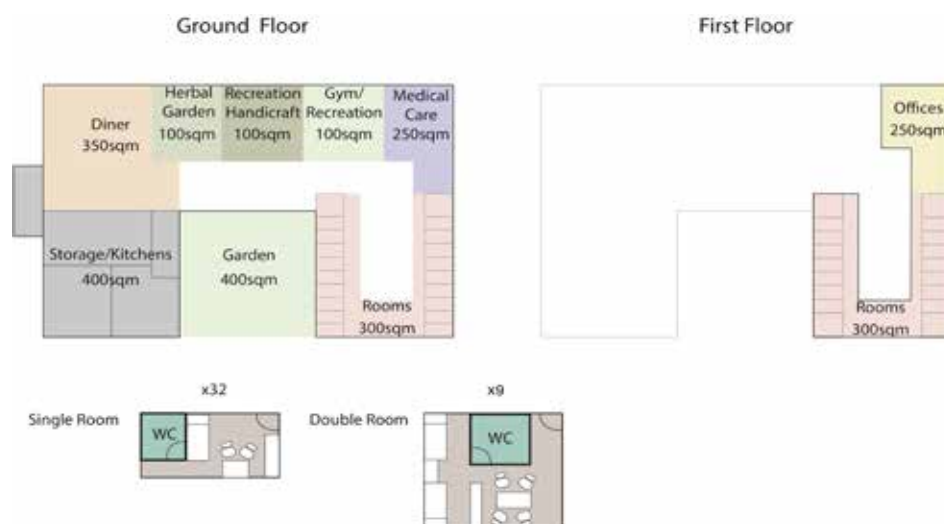
Εικόνα 1. Κάτοψη και Σχεδιασμός Μονάδας (Παρασκευόπουλος 2017).
